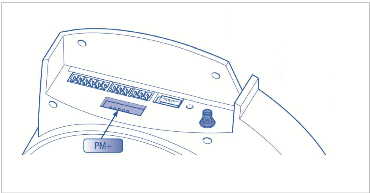
PM+ Schnittstelle bei einem Solar-Log 1000 PM GPRS
