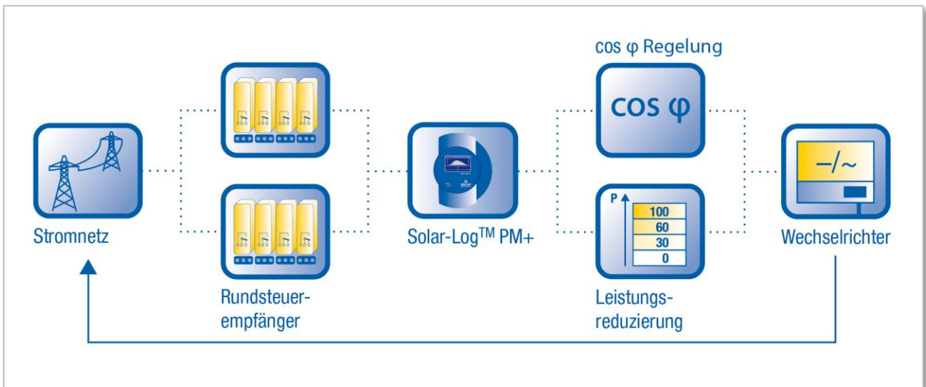
Grundsätzlicher Aufbau Einspeisemanagement
