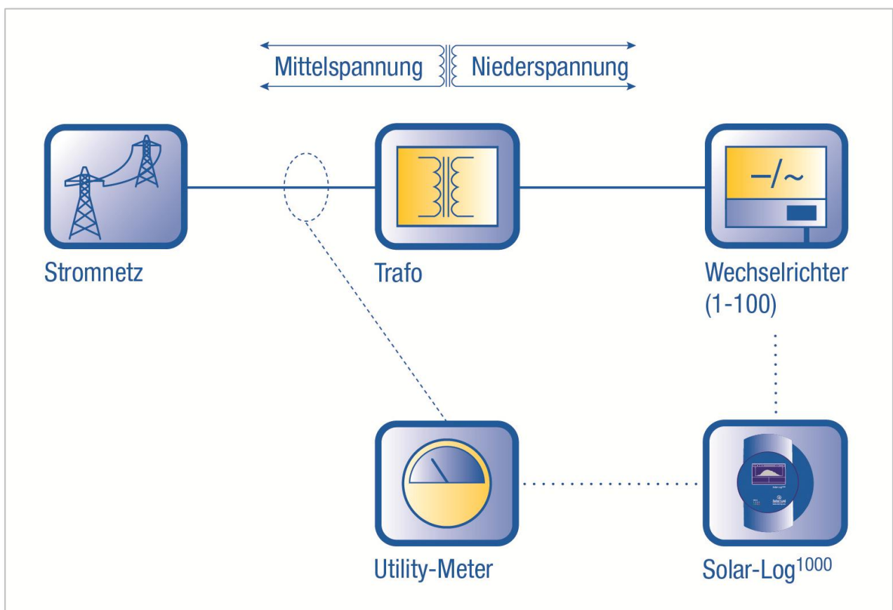
Aufbau variable Blindleistungsbereitstellung per Q(U) Funktion
